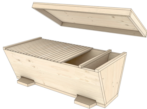
Modell einer „Topbar Hive“
